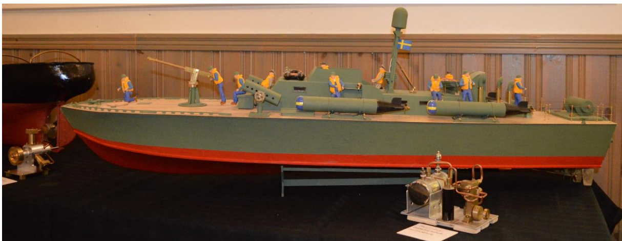
Amerikansk torpedbåt med svenska nationsbeteckningar. I förgrunden en ångmaskin.
